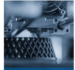
Fabricación aditiva
